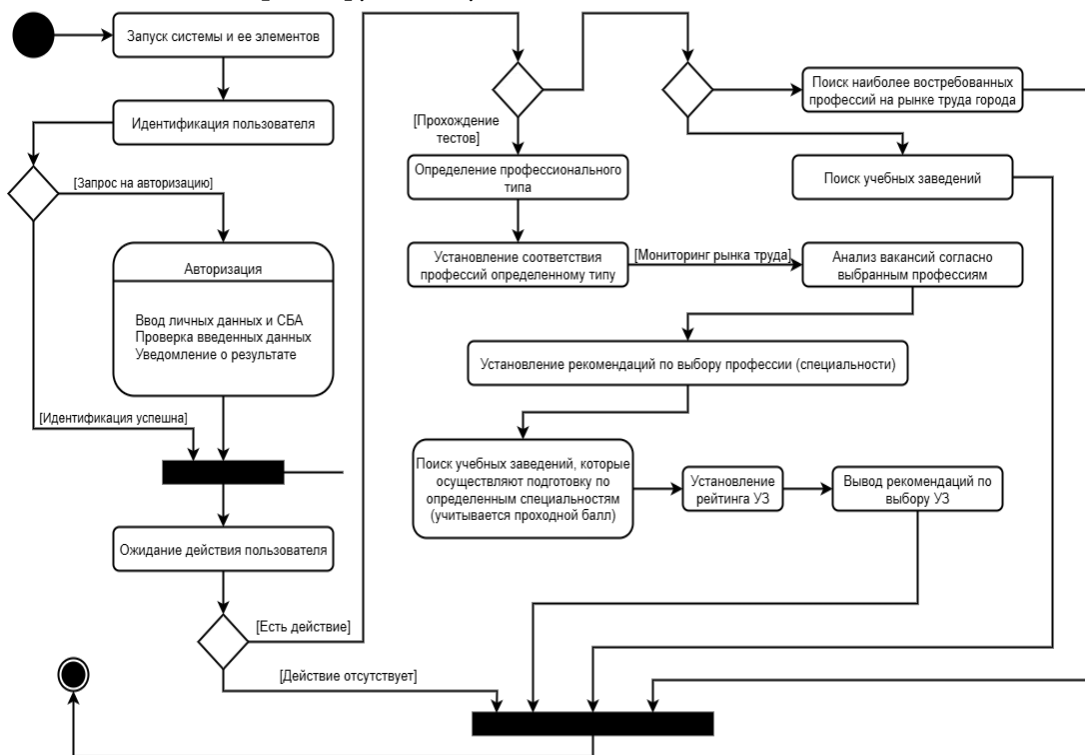
Рис. 6. Алгоритм функционирования ПАК.
