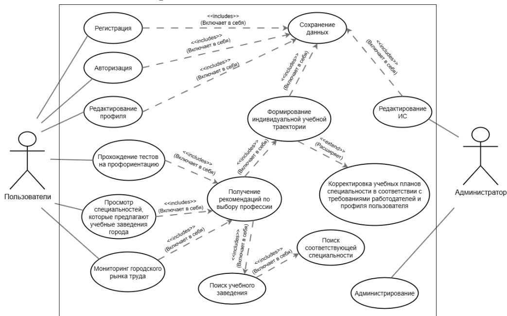
Рис. 4. Диаграмма вариантов использования программно-алгоритмического комплекса сопровождения подготовки специалистов.
