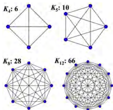
Рис. 2.1. Полные графы.
