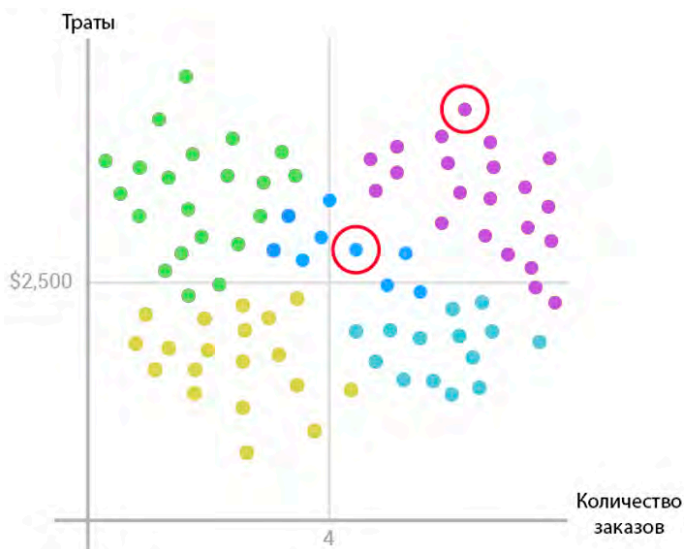
Рис. 2. Кластерный анализ.
