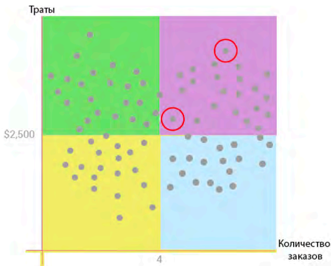
Рис. 1. Пороговая сегментация.
