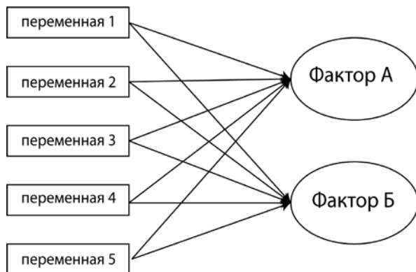
Рис. 3. Факторный анализ.
