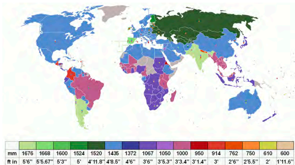
Рис. 1. Железнодорожная колея в разных странах мира.
