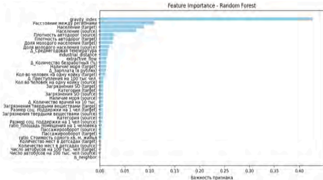
Рис. 2. Важность признаков.
